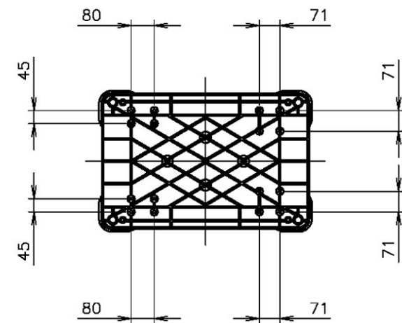
裏面詳細図
